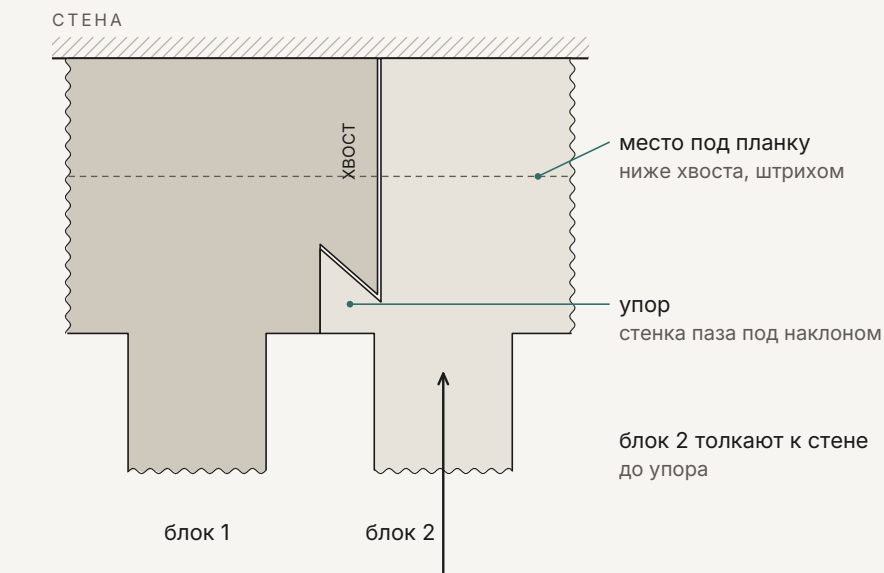
ВИД СВЕРХУ · РАЗРЕЗ ПО ХВОСТУ
