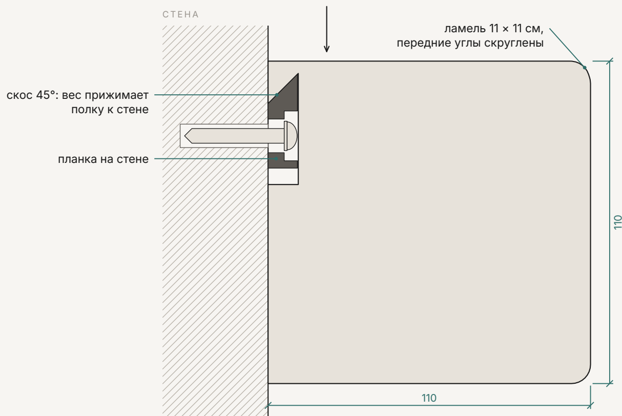
РАЗРЕЗ ПО ЛАМЕЛИ · РАЗМЕРЫ В ММ
